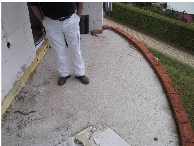
Neubau Balkonabdichtung: Abdichtung sowie Belag
